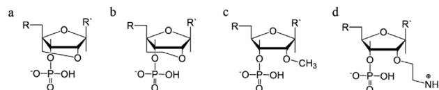
Fig. 12 Sugar backbone modifications. (a) LNA, (b) ENA, (c) 2'-OMe, (d) 2'-AE.
