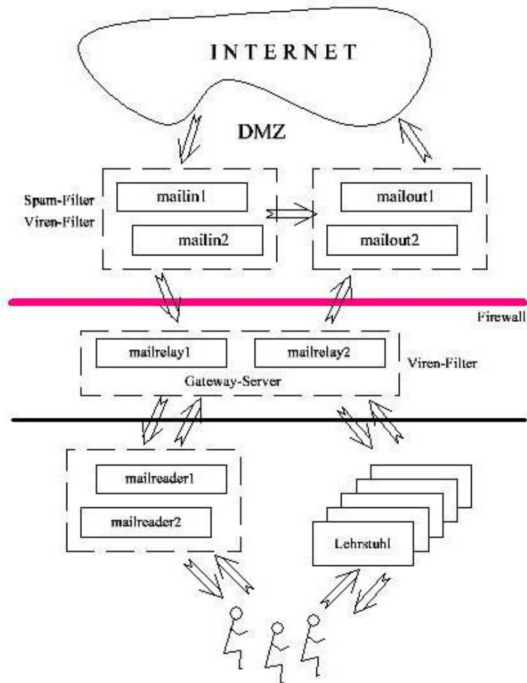
Zentrale E-Mail-Infrastruktur der Informatik
