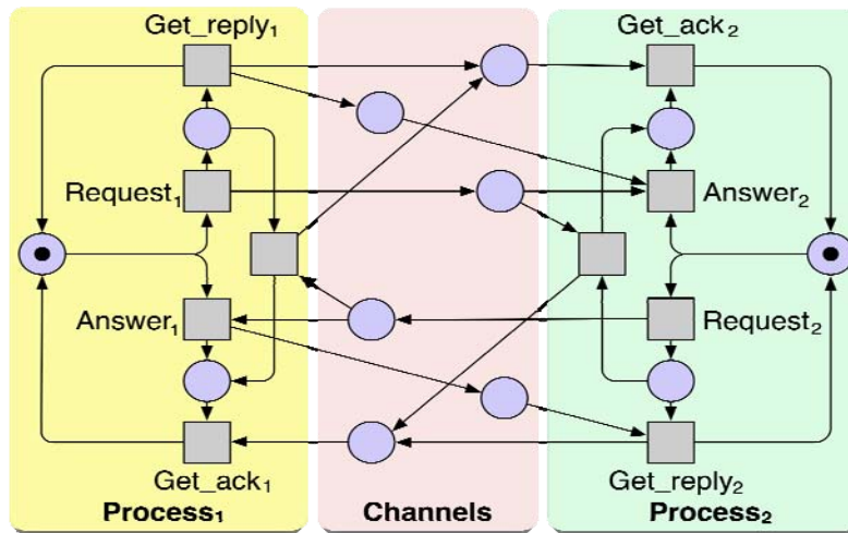
Petrietzmodell eines einfachen Kommunikationsprotokolls
