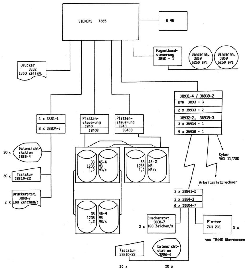
Teilsystem A: Siemens 7.860-Konfiguration
