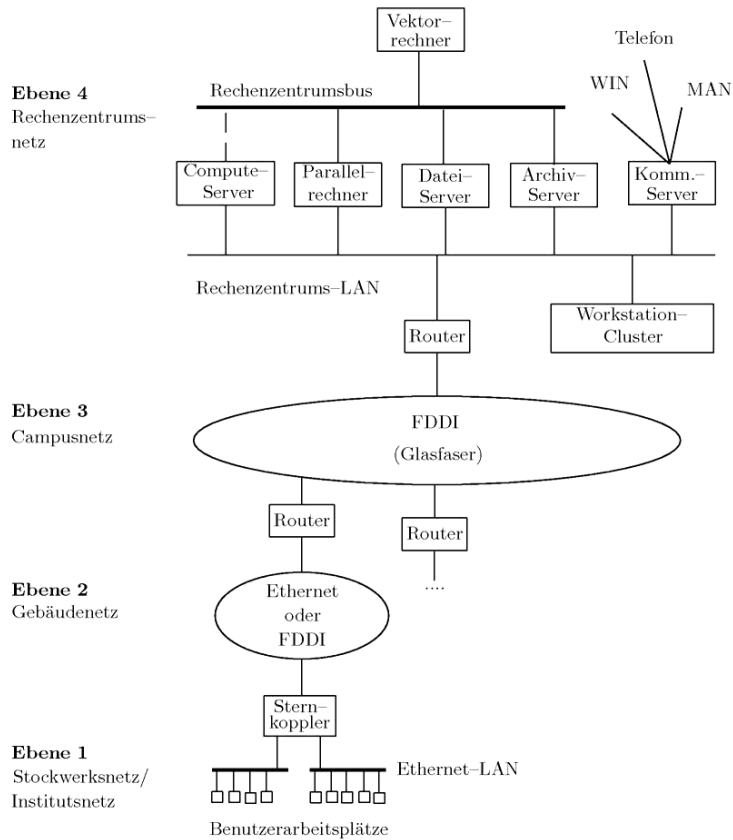
Vernetzungsstruktur von WAP
