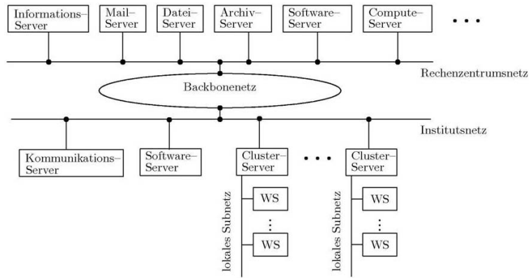
Kooperatives Versorgungskonzept
