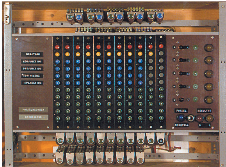
Formelgesteuerte Rechenmaschine für Aussagenlogik STANISLAUS
