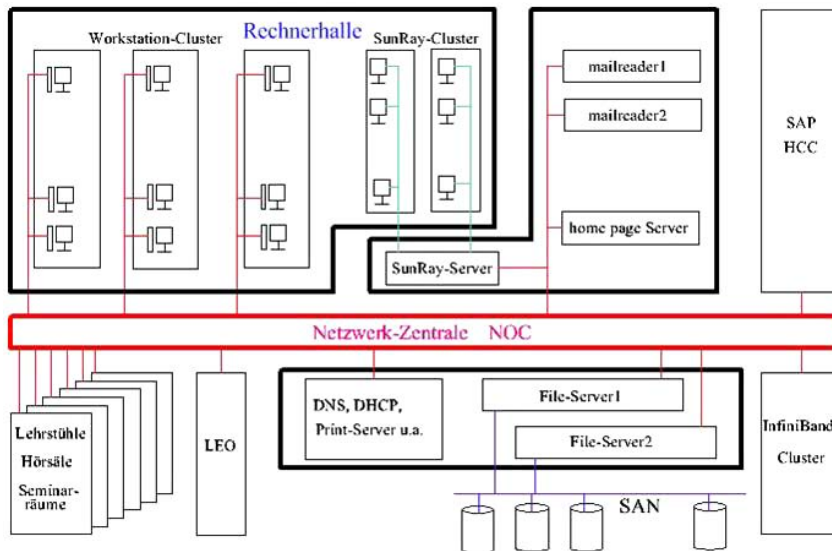
Netzübersicht Garching
