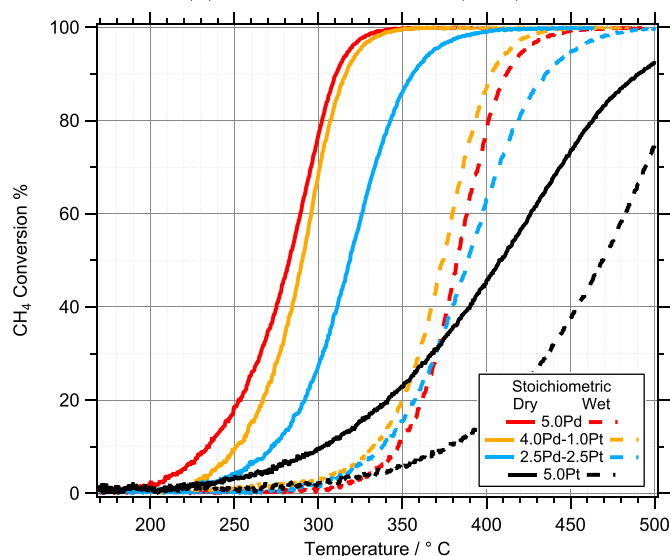
(b) \text{CH}_4:\text{O}_2:\text{H}_2\text{O} 1:2(:100)
